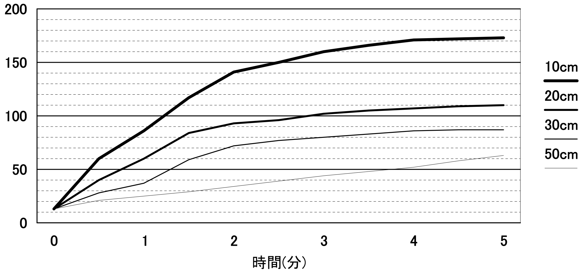
CBH-2022温度性能グラフ(中心部測定) ファン無
