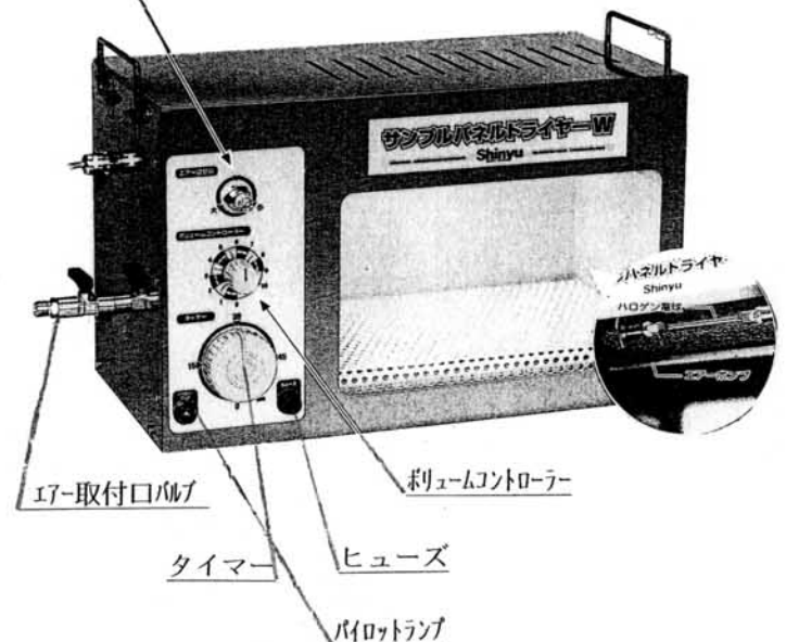
エアー調整器
